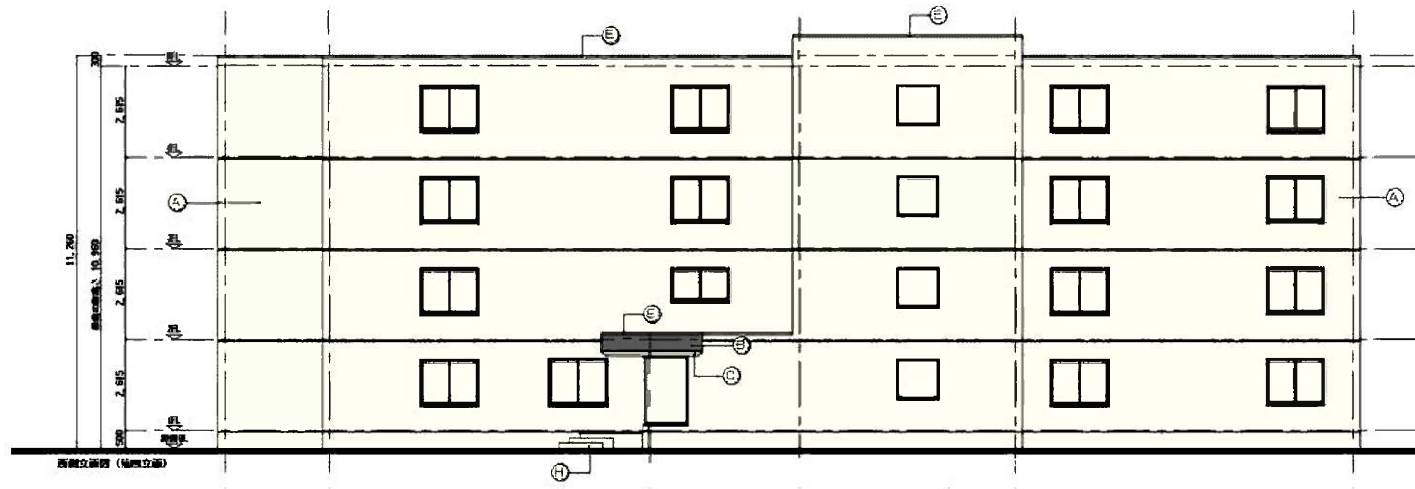
西側立面图
