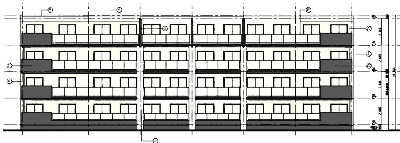
東側立面图
