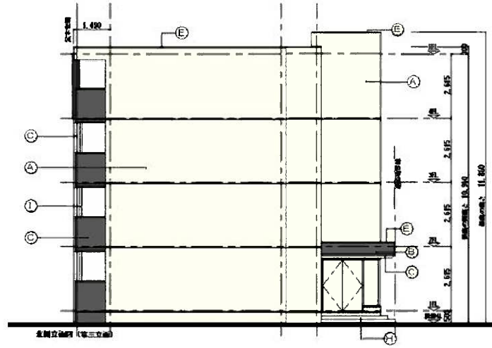
北側立面图
